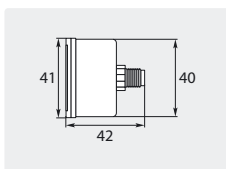
∅ 40 mm. 1/8" M. Boîtier PVC. Entrée latérale
